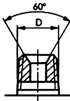
Amerikanisches Standardaußen- gewinde NPT
